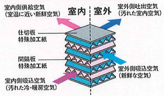
■ロスナイエレメント(熱交換器)における熱交換イメージ
